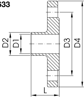
Vorschweißflansch welding neck flange
