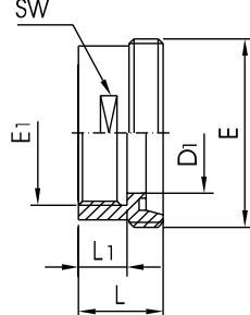
Gewinde-Aufschraubstutzen female part adapter
