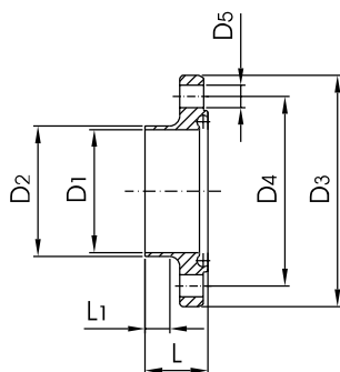
Nutflansch Zoll (kurz) notch flange inch (short)
