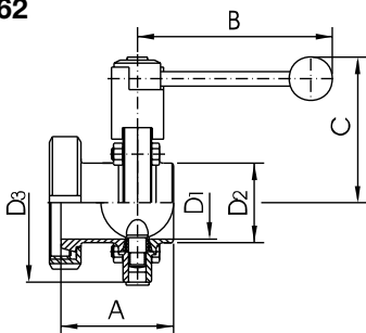
Scheibenventil DIN-KS btf. valve-DIN-liner/welding end
