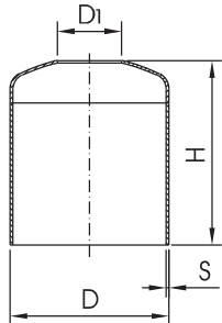
Glocke zum Anschweißen bell for tubes
